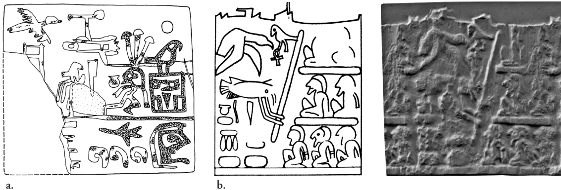
FIG. 8. Représentations du roi sous les traits d’un poisson-chat agissant. a. Étiquette en ivoire, Oum el-Qaab, cimetière B, à proximité de la tombe B16-2 – règne de Nârmer (d’après G. Dreyer et al. , « Umm el-Qaab. Nachuntersuchungen im frühzeitlichen Königsfriedhof. 9./10. Vorbericht », MDAIK 54, 1998, p. 139, fig. 29) ; b. Cylindre en ivoire, grand dépôt de Hiérakonpolis, Ashmolean Museum E.3915 – empreinte et dessin (d’après P. Kaplony, Die Inschriften der ägyptischen Frühzeit III, ÄgAbh 8, Wiesbaden, 1963, fig. 5).
